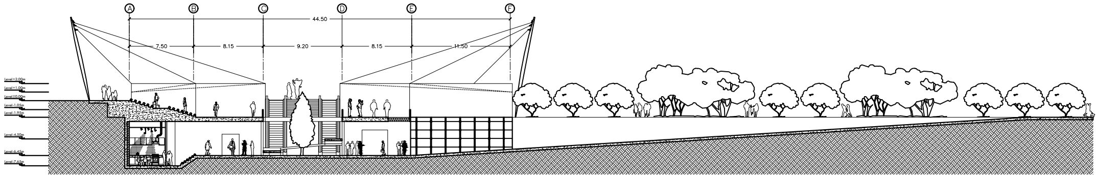
02 Section A-A Sc: 1/100
