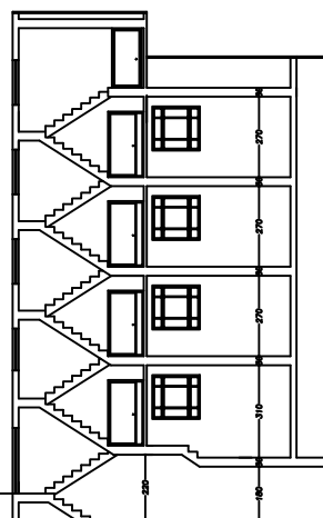
SECTION A-A SC. 1:100
